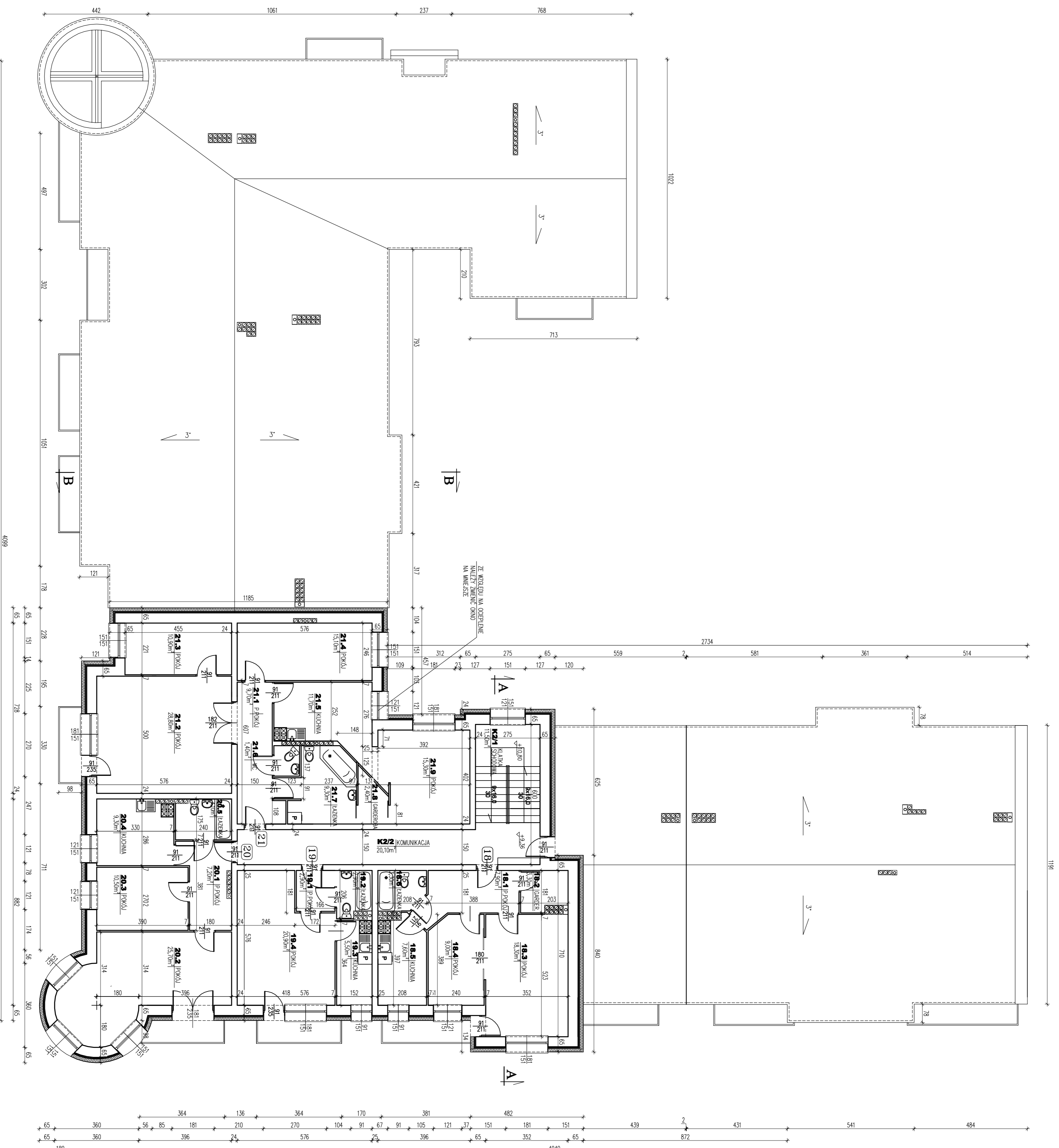
RZUT PODDASZA 1:100
