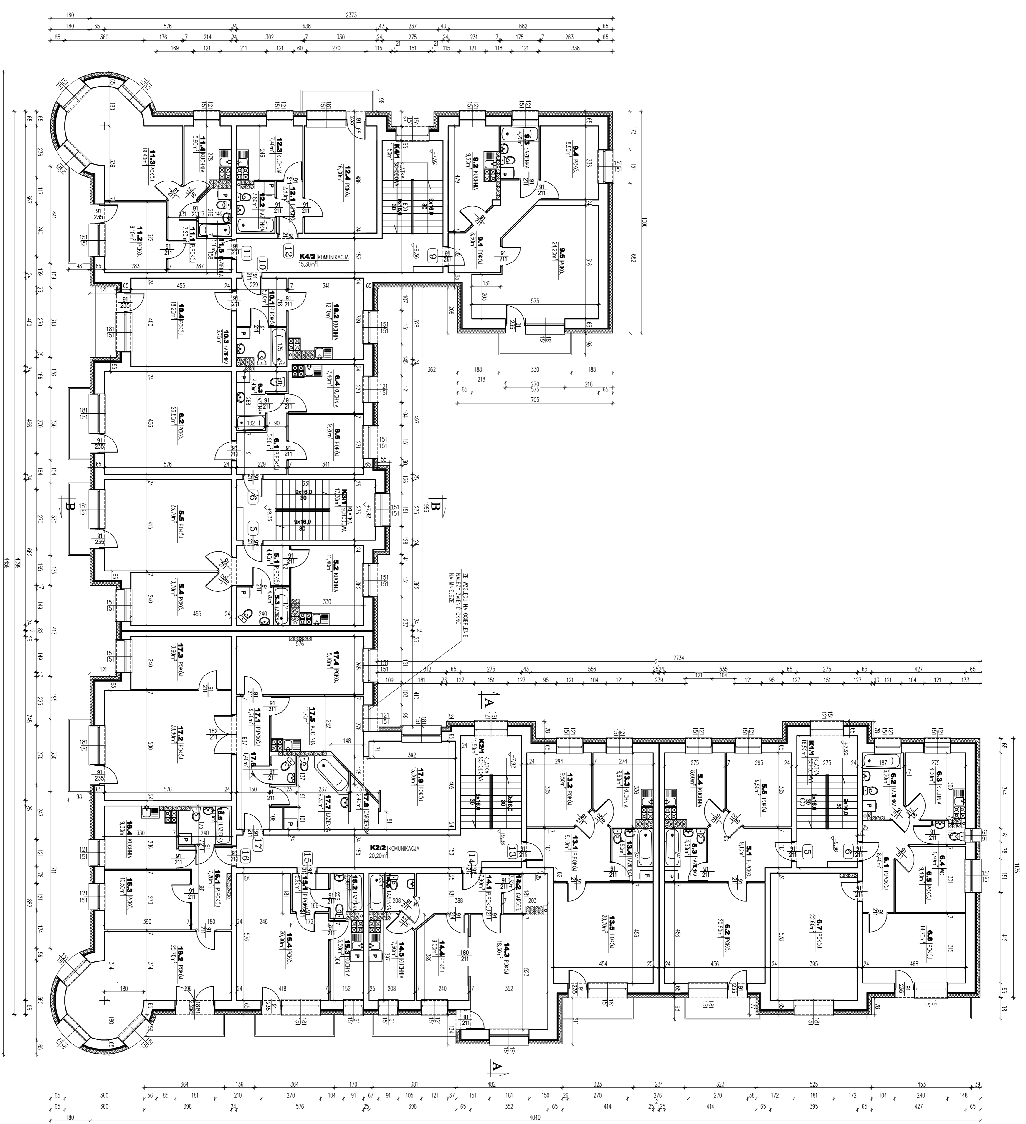
RZUT III PIĘTRA 1:100
