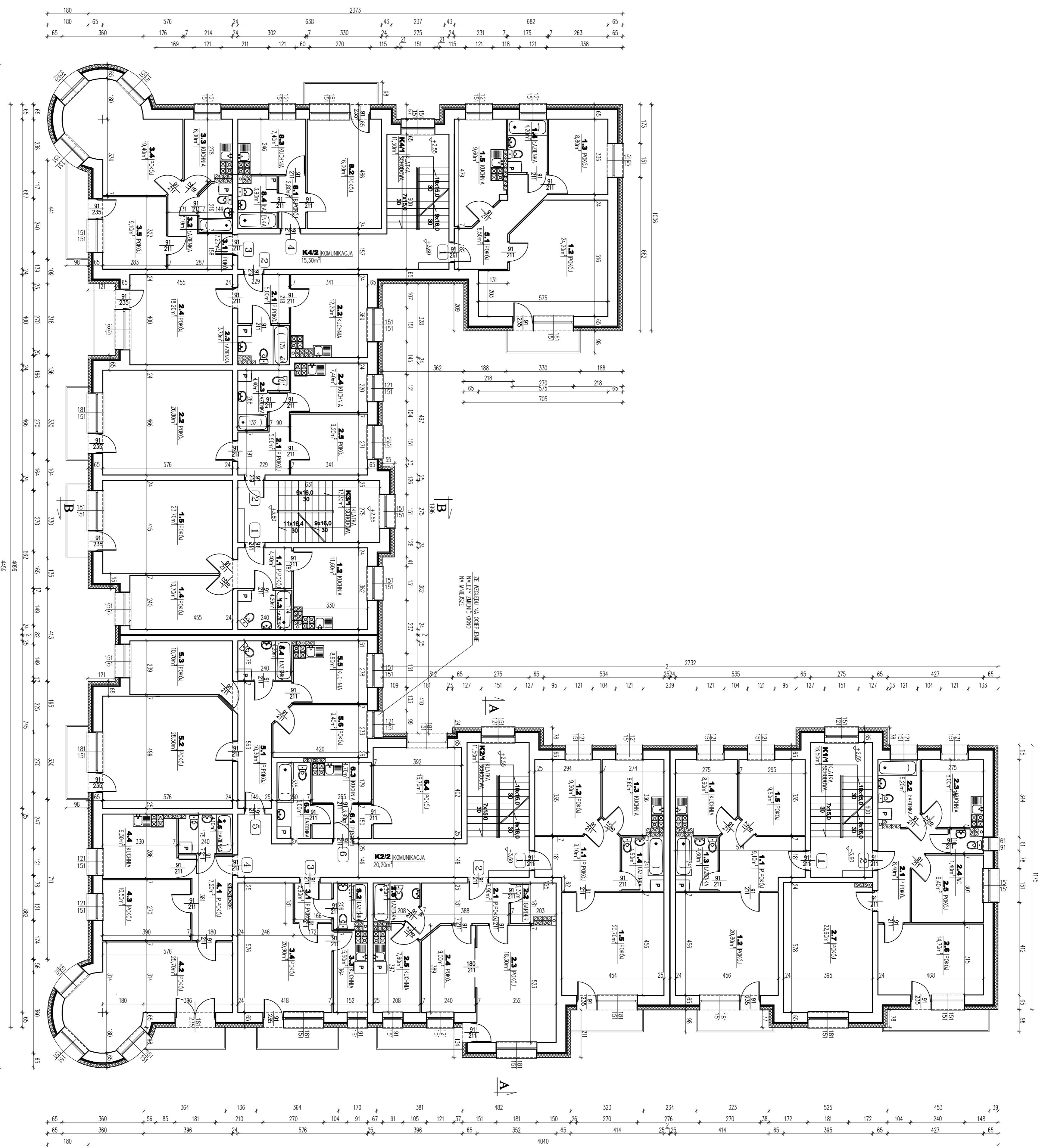
RZUT I PIĘTRA 1:100
